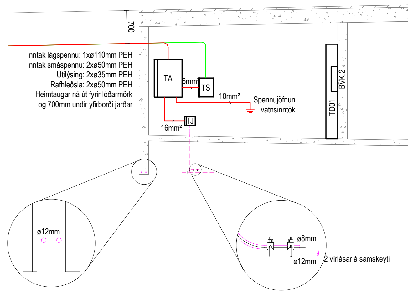
Snið í inntök 1 : 50
